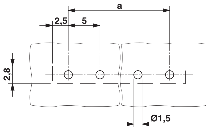
Bohrplan/Lötpadgeometrie
