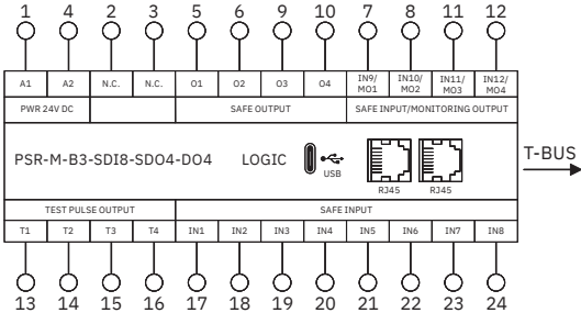
Schéma fonctionnel
