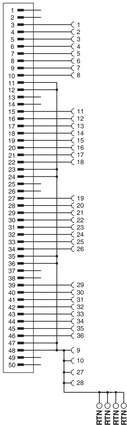
Schaltplan
