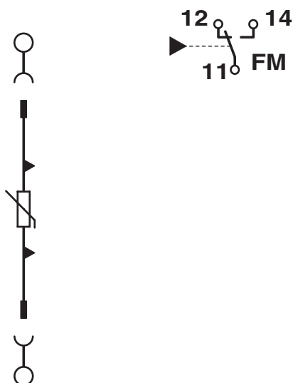
Diagrama eléctrico
