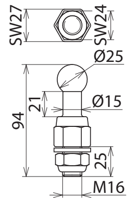
Maßbild KFP 25 M16 25 SKM
