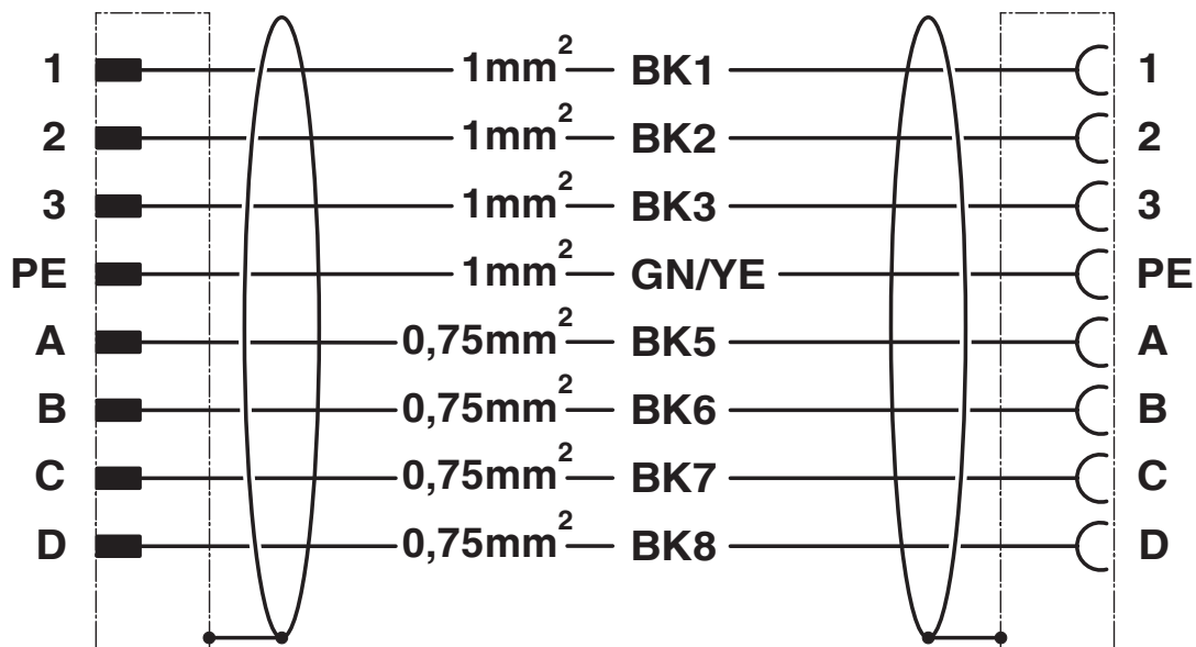
Diagrama eléctrico
