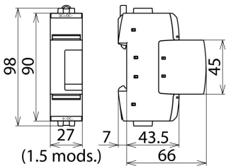
Dimensiones del DG SE DC 900
