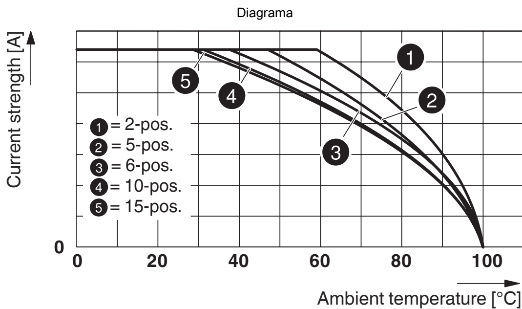
Diagrama eléctrico
