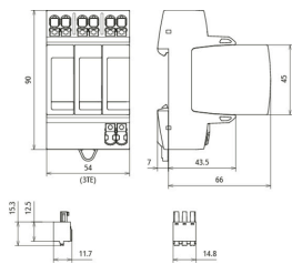
Dimensioni DG MP YPV 1200 FM
