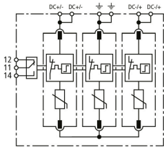
Schema di circuito basilare DG MP YPV 1200 FM
