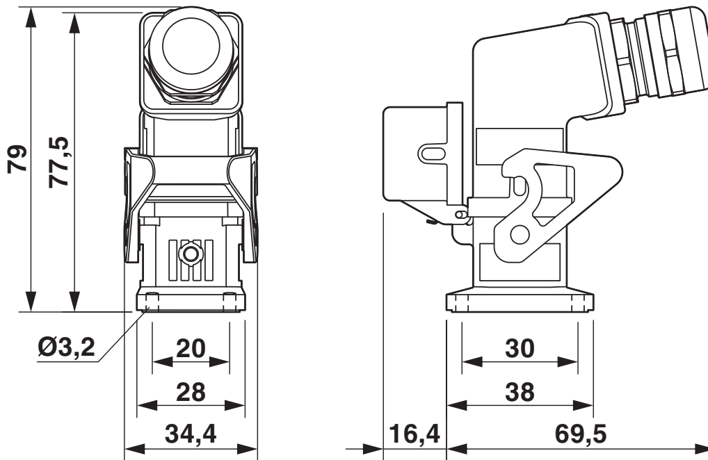
Maßzeichnung
