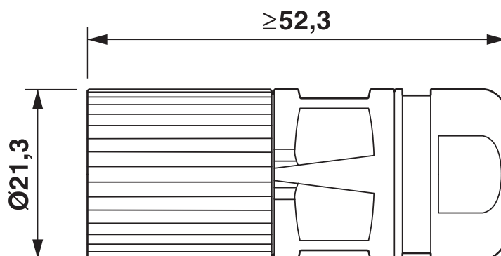
Maßzeichnung
