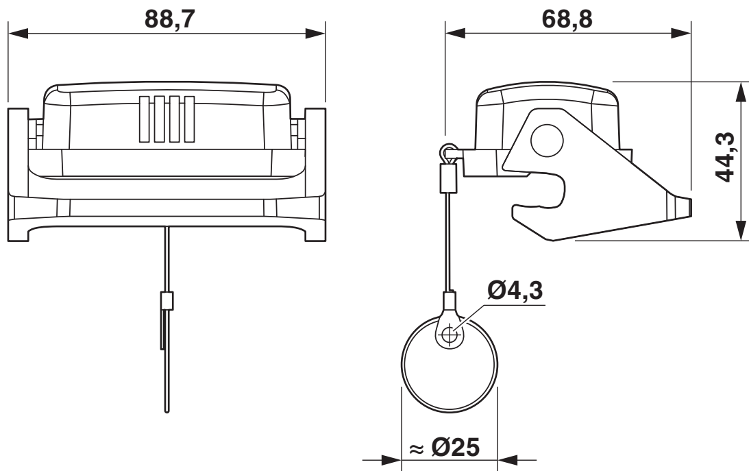
Maßzeichnung
