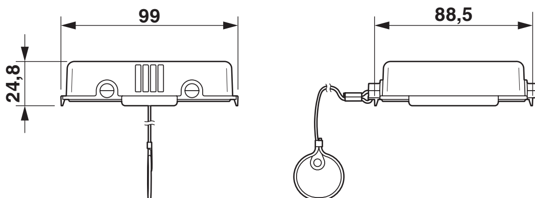
Dessin coté
