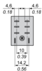
Stecker-Seitenansicht
