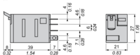
Stecker-Seitenansicht
