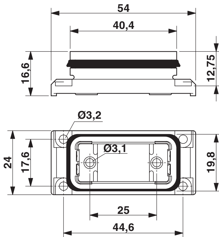
Dessin coté
