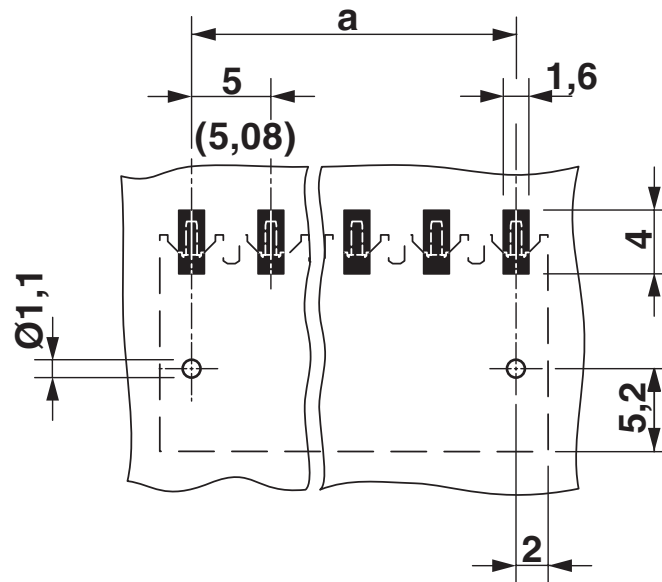
Bohrplan/Lötpadgeometrie
