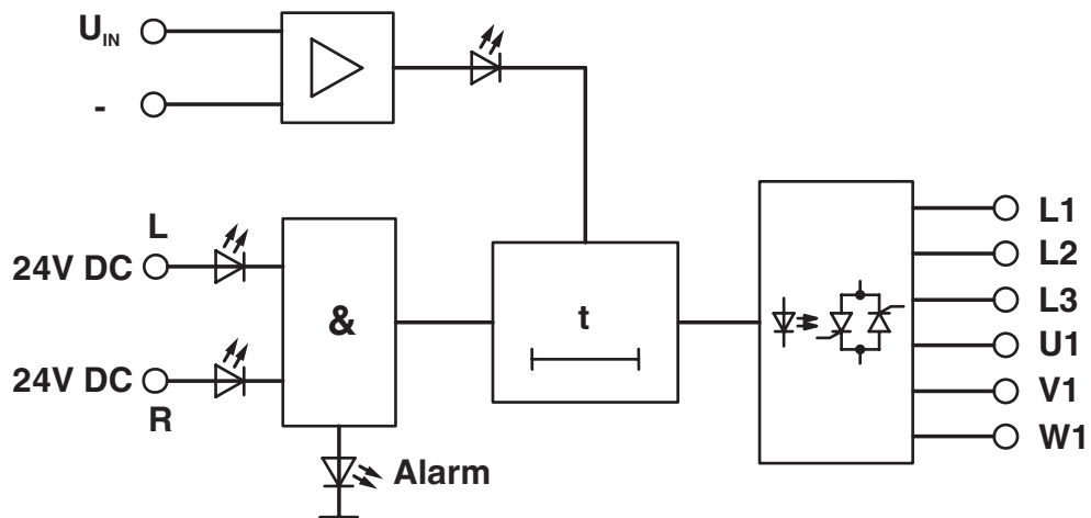
Blockschaltbild
