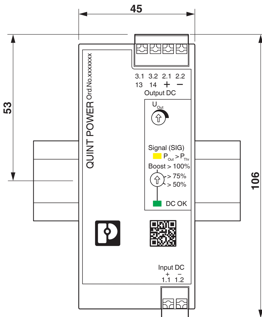
Dessin coté
