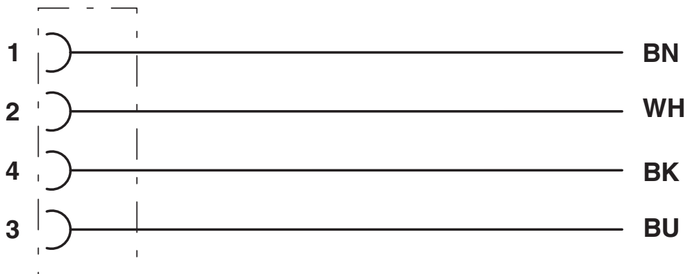
Diagrama eléctrico
