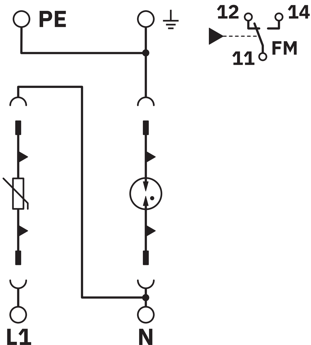
Diagrama eléctrico
