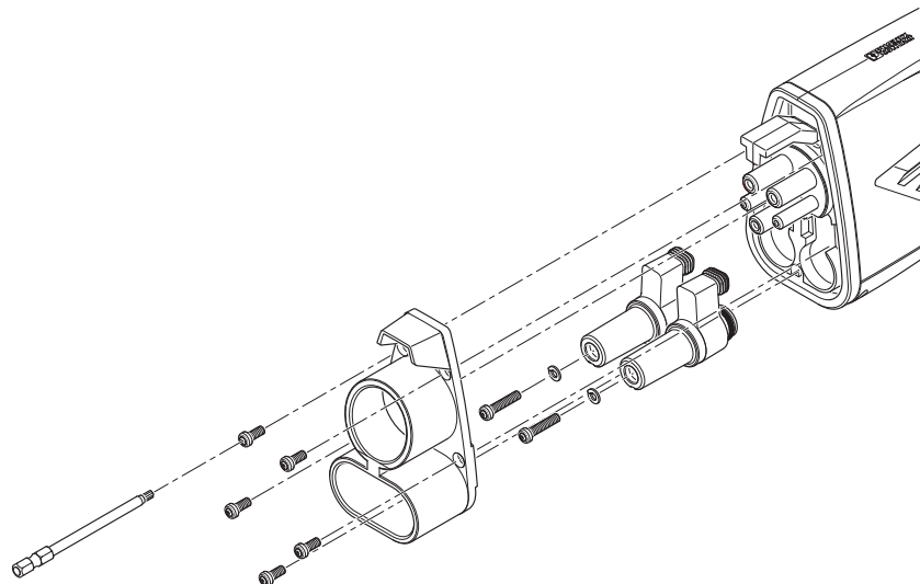
Plano esquemático
