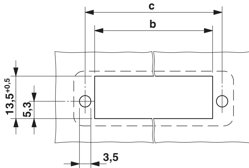
Bohrplan/Lötpadgeometrie
