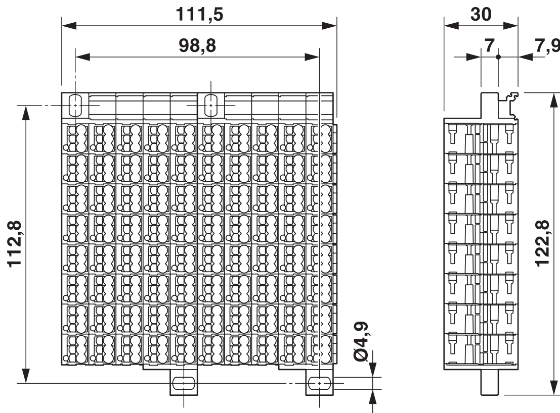
Dessin coté
