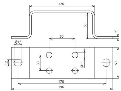
Maßbild ES 2X2 ASB11 V2A
