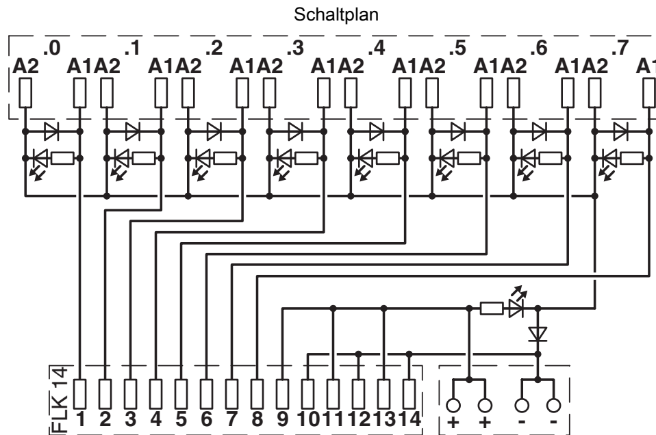
Anschlussbild RIF-1-V8/PT/FLK14/OUT
