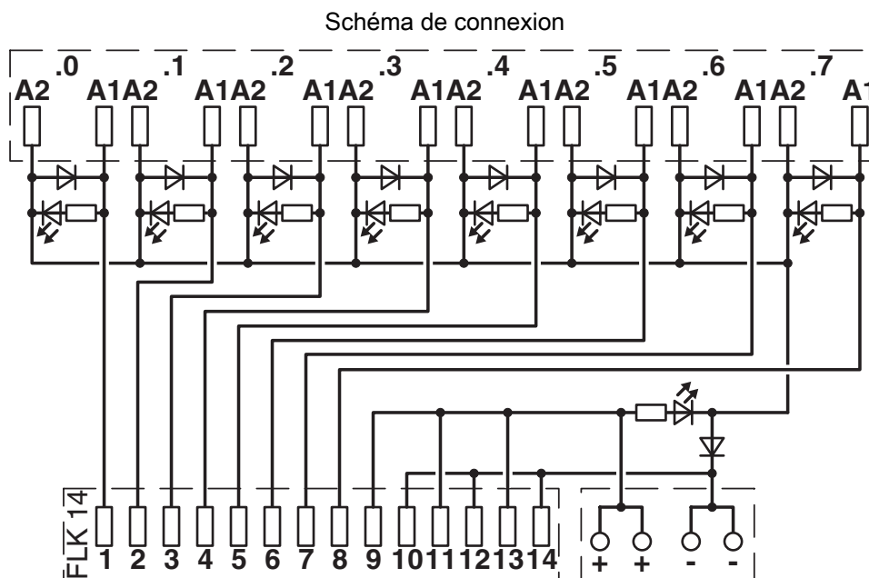
Schéma des connexions RIF-1-V8/PT/FLK14/OUT
