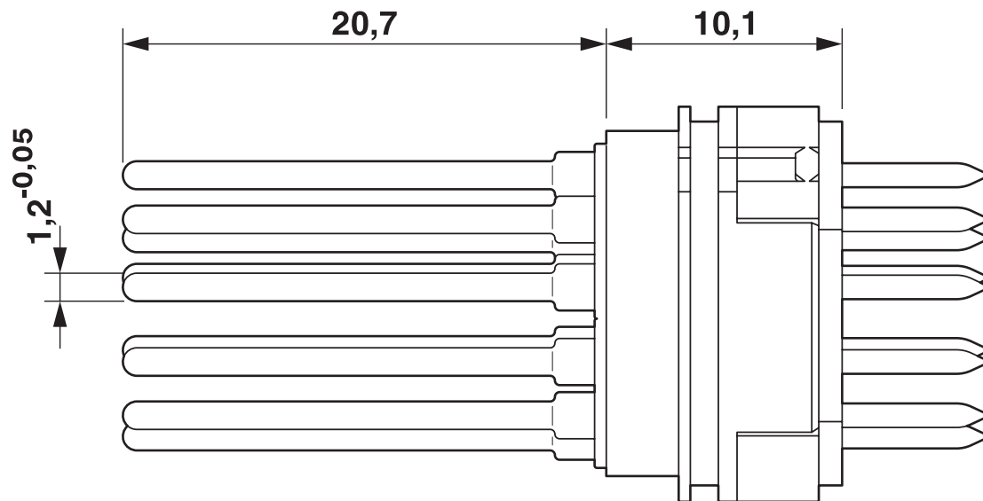
Maßzeichnung
