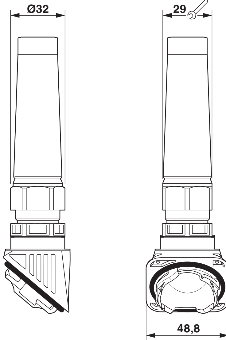
Dessin coté
