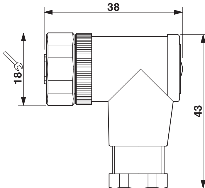
Maßzeichnung
