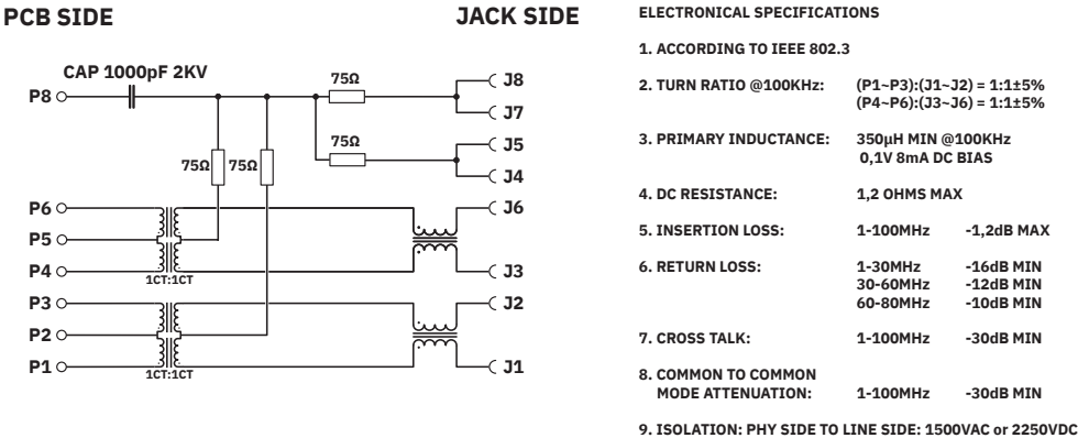
Diagrama eléctrico
