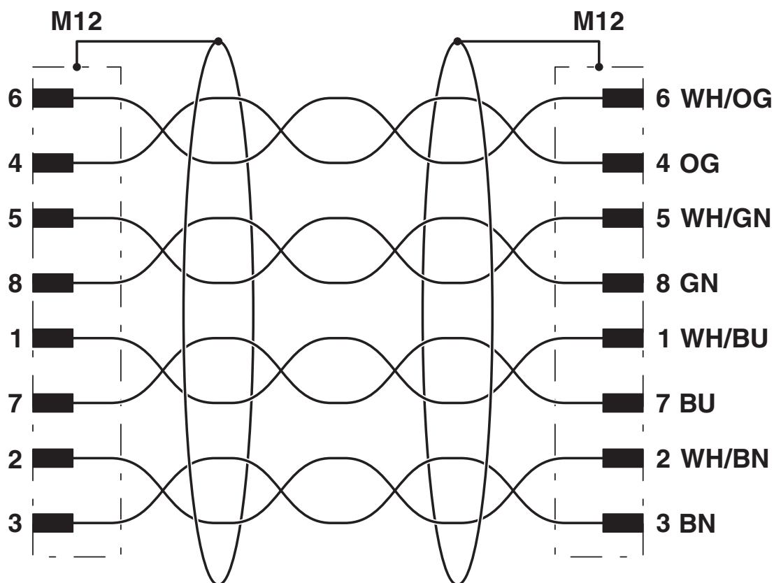
Diagrama eléctrico
