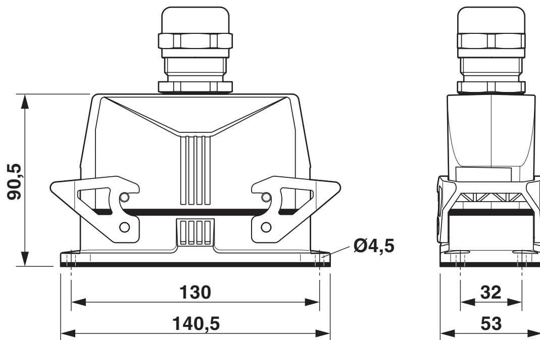
Maßzeichnung
