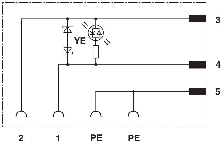
Schaltplan
