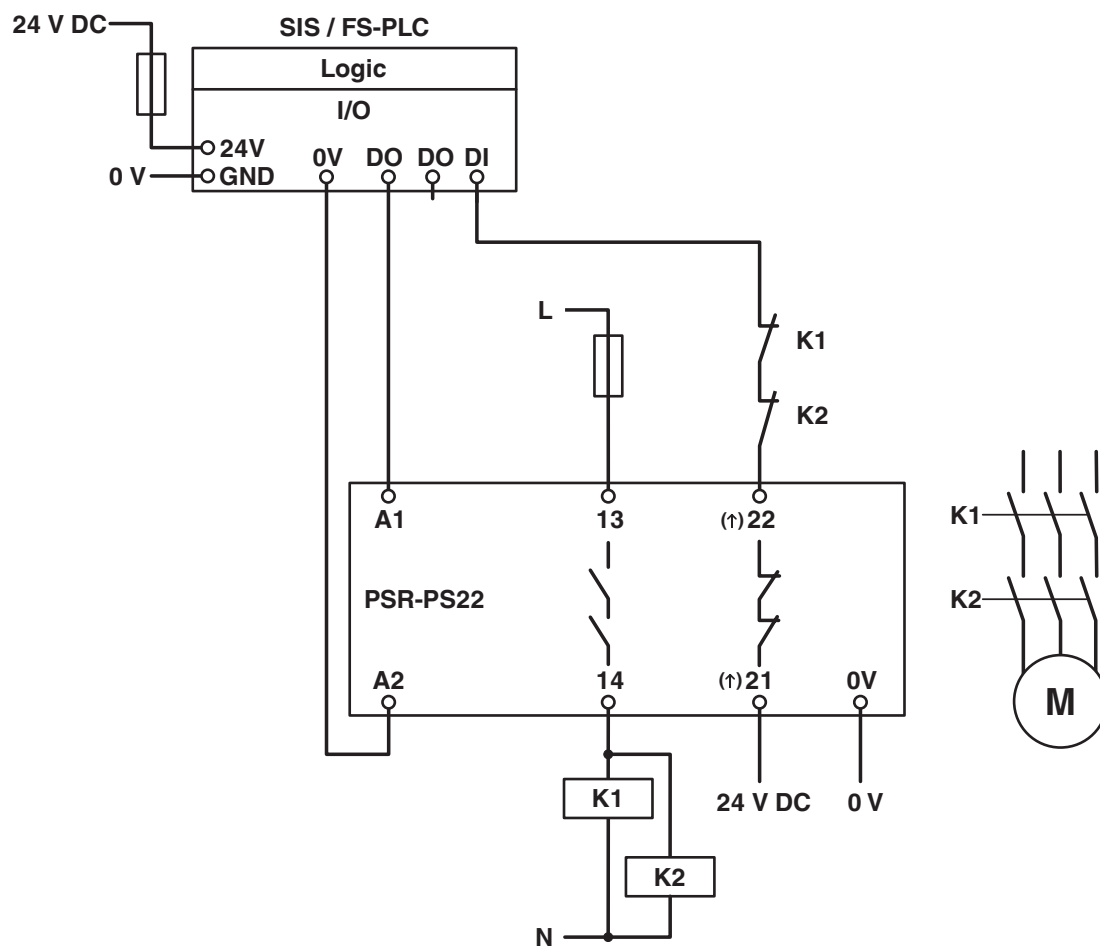
Diagrama eléctrico
