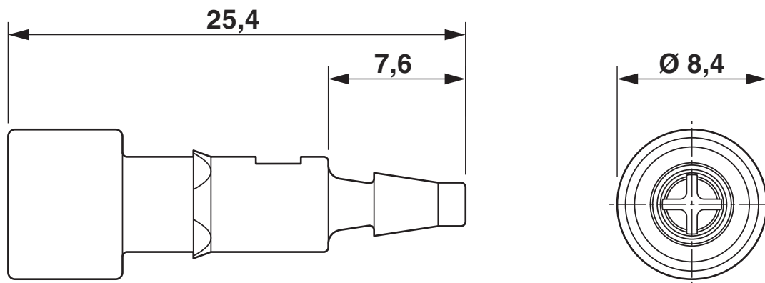
Maßzeichnung
