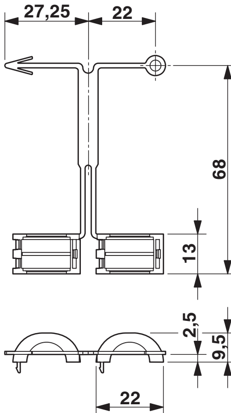
Maßzeichnung
