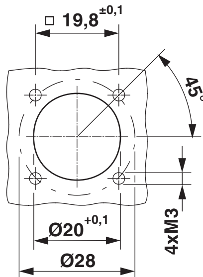
Schemazeichnung
