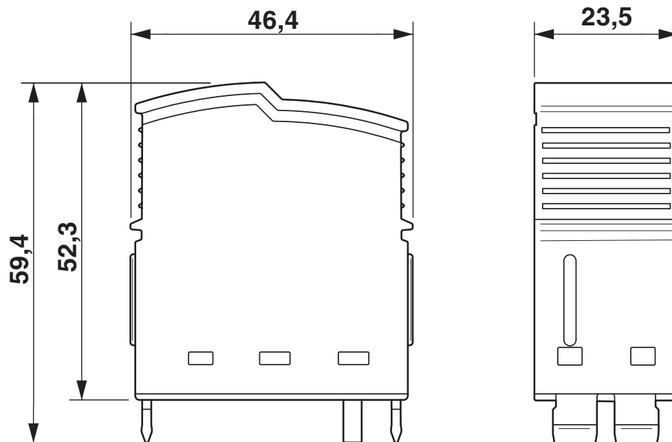
Dessin coté
