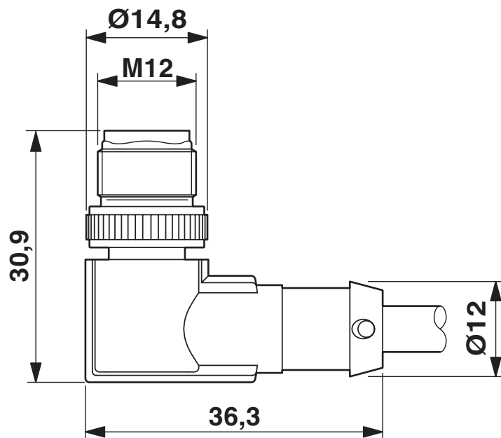
Maßzeichnung
