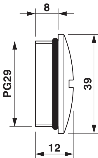
Esquema de dimensiones
