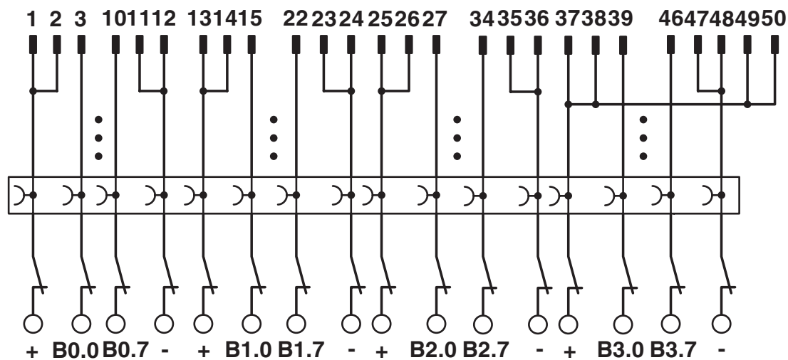
Esquema de conexiones FLKM 50/KDS3-MT/PPA/PLC
