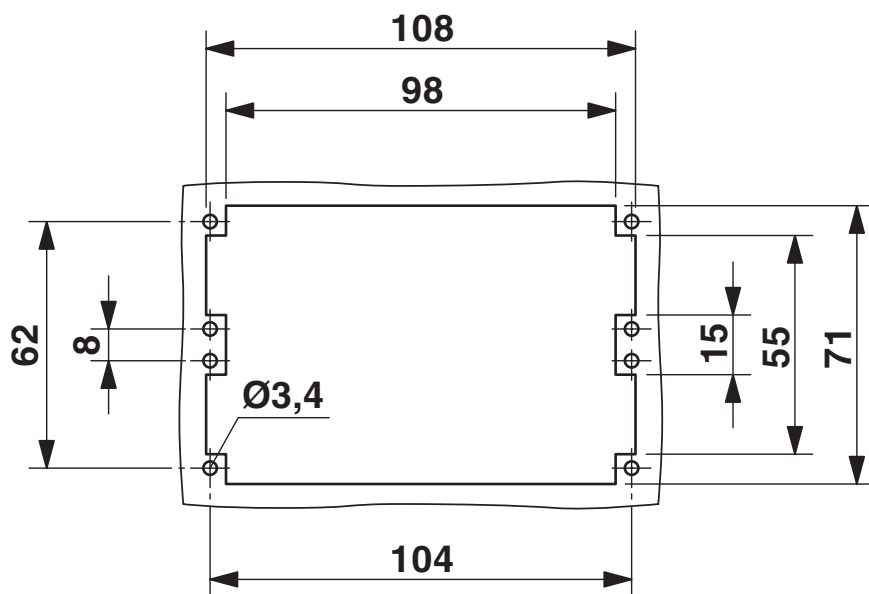
Dessin coté
