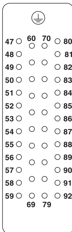
Dessin schématique
