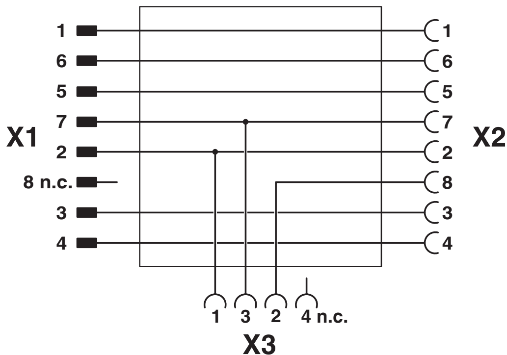
Diagrama eléctrico
