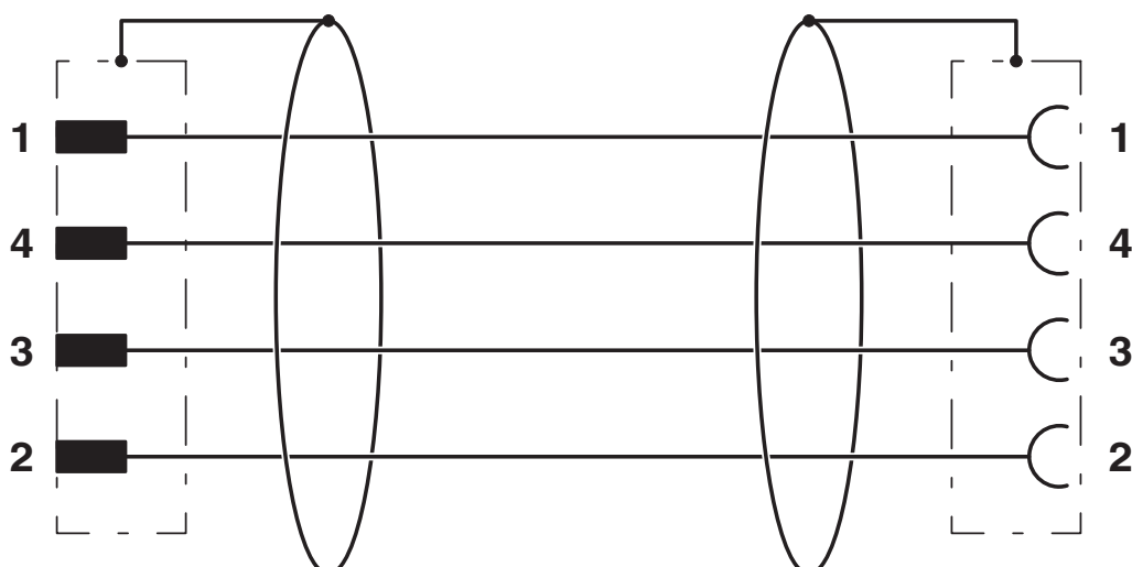
Diagrama eléctrico
