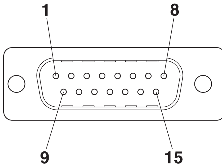
Schemazeichnung
