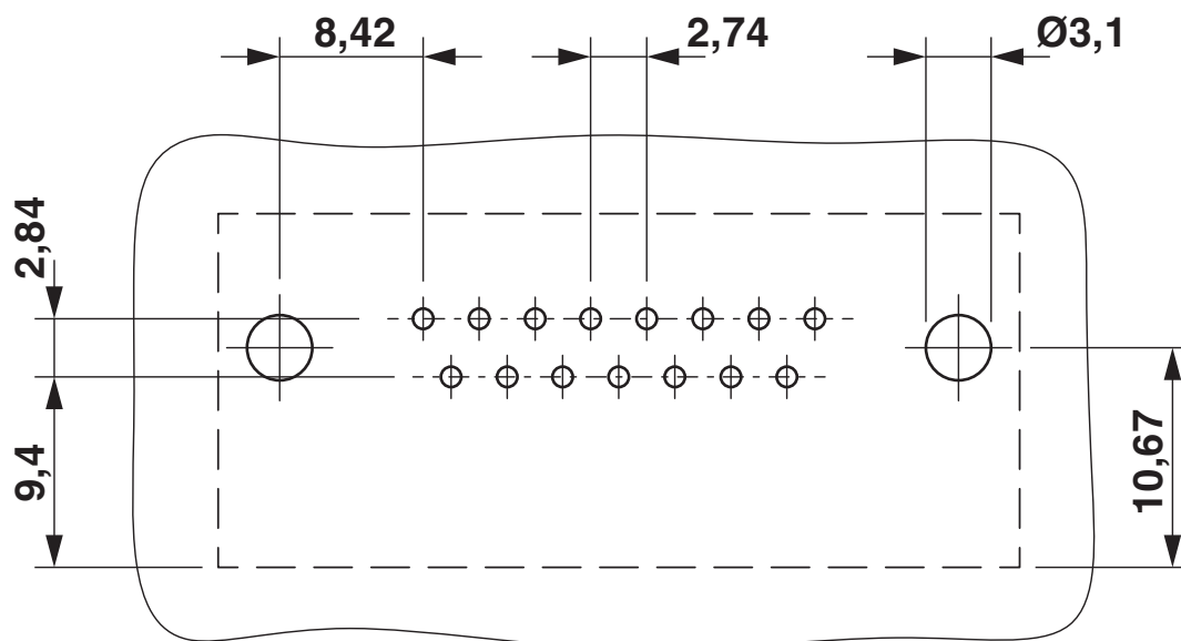
Bohrplan/Lötpadgeometrie
