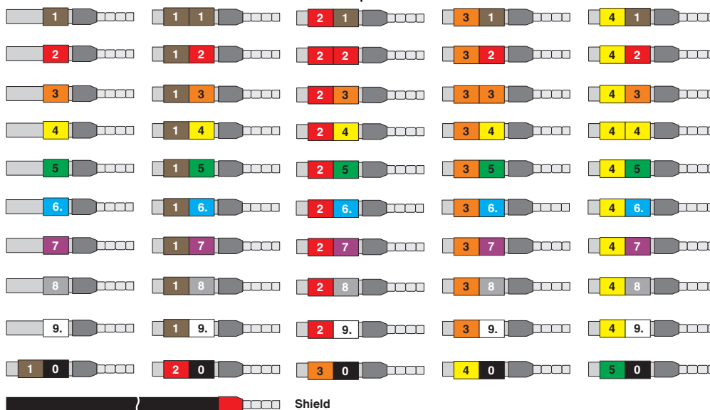
Plano esquemático
