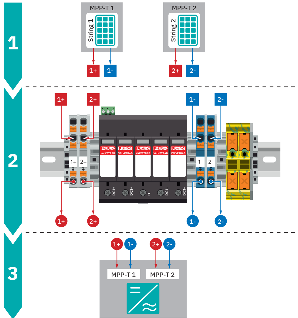
Schematische Applikationszeichnung
