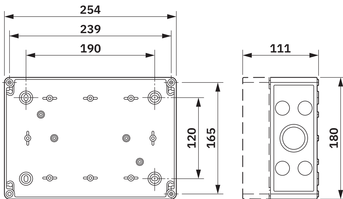
Dimensions du boîtier
