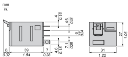
Stecker-Seitenansicht
