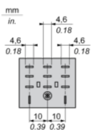
Stecker-Seitenansicht
