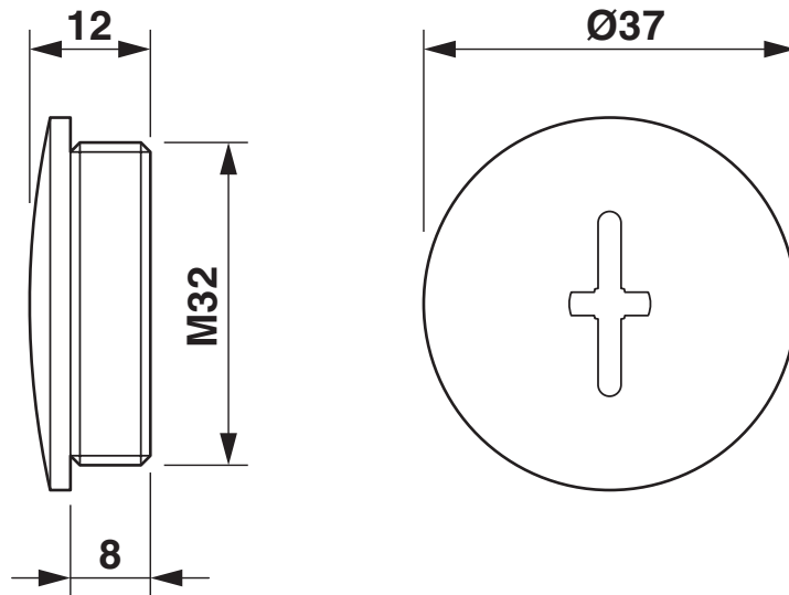
Maßzeichnung
